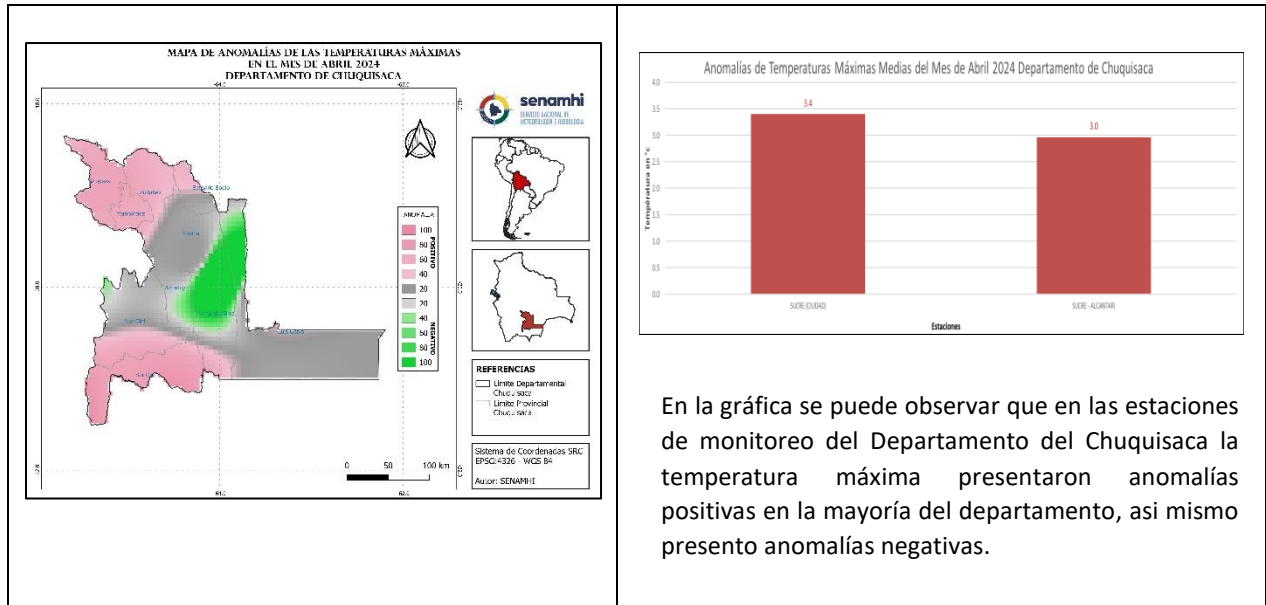
Ilustración 8 Mapa de Anomalia de Temperatura Máxima para el mes de abril 2024
