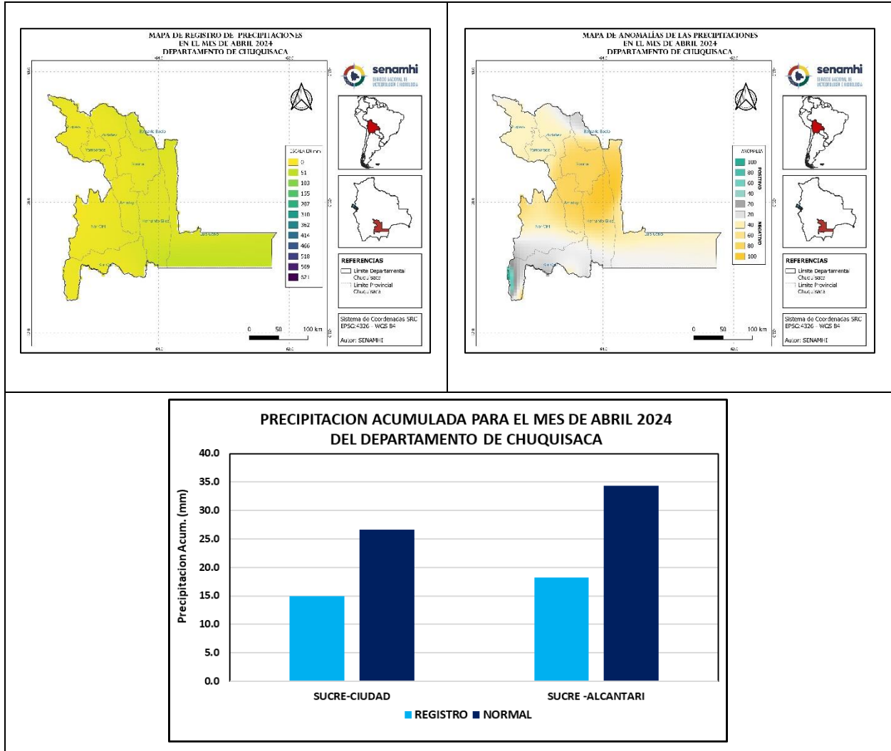
Ilustración 5 Mapa y Grafica de Registro de Precipitaciones para el mes de abril 2024
