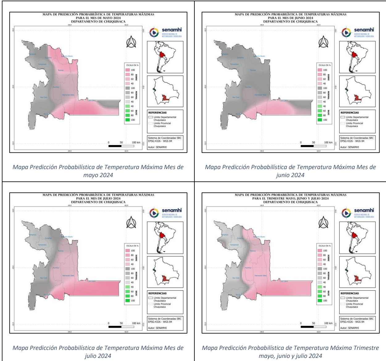
Ilustración 13 Mapas de Predicción Probabilística de las Temperaturas Máximas Medias para el trimestre MJJ 2024
