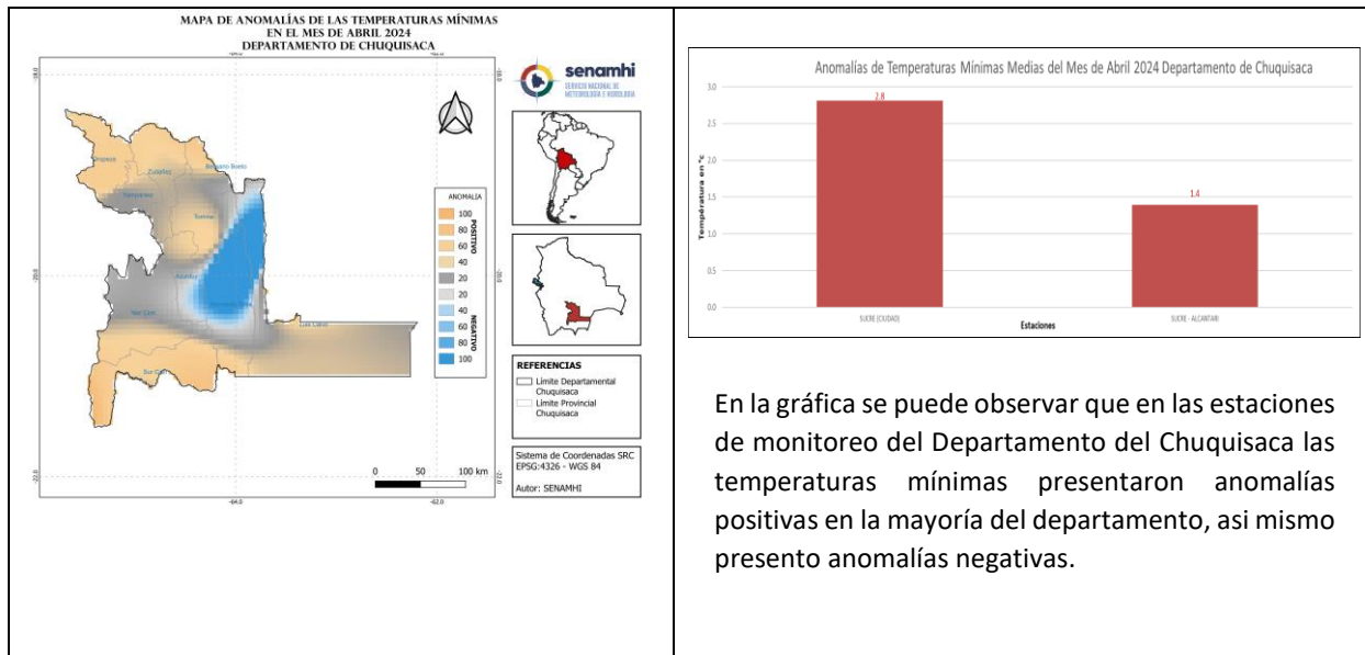
Ilustración 11 Mapa de Anomalía de Temperatura Mínima para el mes de marzo 2024
