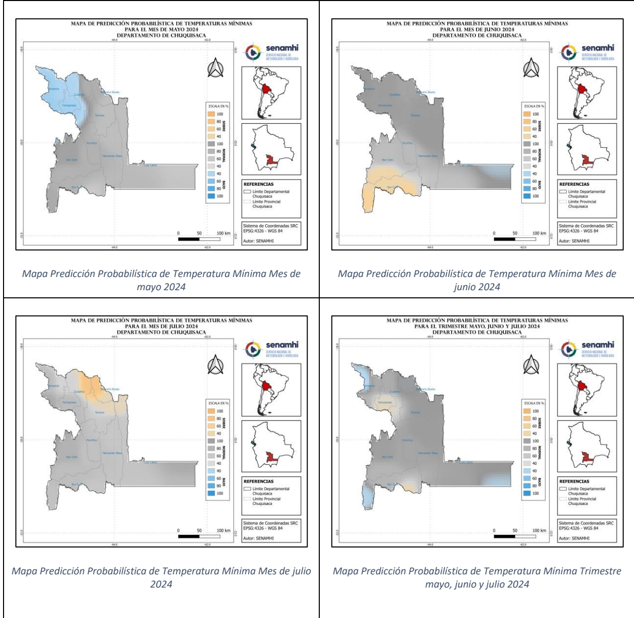
Ilustración 14 Mapas de Predicción Probabilística de las Temperaturas Mínimas Medias para el trimestre MJJ 2024
