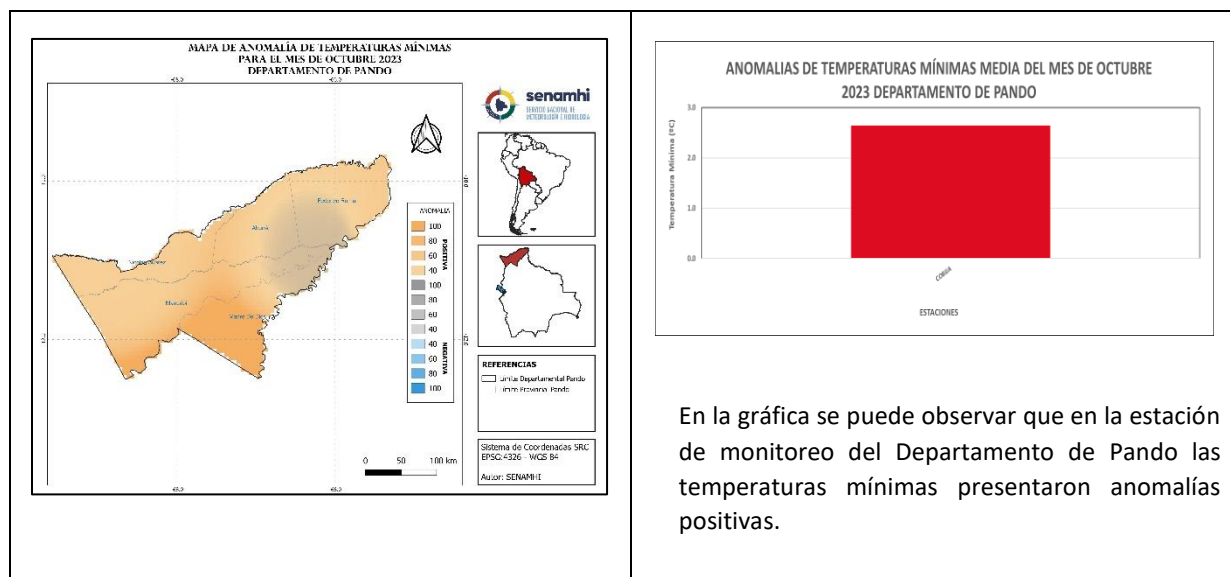
Ilustración 7 Mapa de Anomalía de Temperaturas Mínimas para el mes de octubre 2023
