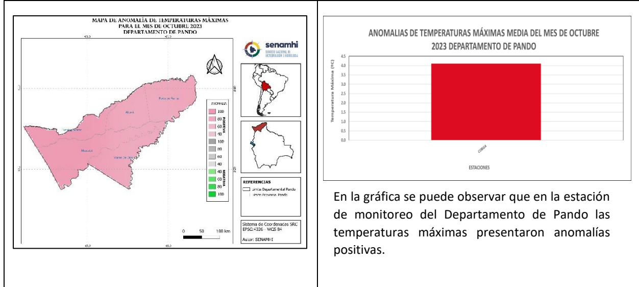
Ilustración 6 Mapa de Anomalia de Temperaturas Máximas para el mes de octubre 2023
