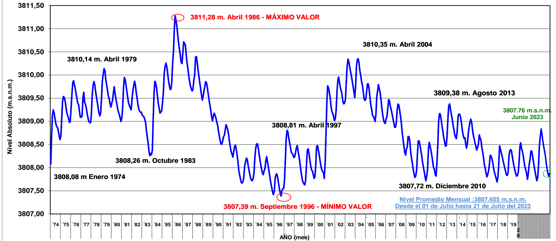
LAGO TITICACA: ESTACIÓN HUATAJATA NIVELES MEDIOS MENSUALES (SERIE 1974 - 2023)
