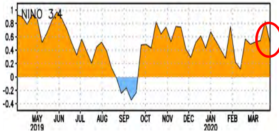
Anomalías de las temperaturas superficiales del océano pacífico (Región 3.4) hasta abril de 2020 Figura 1.
