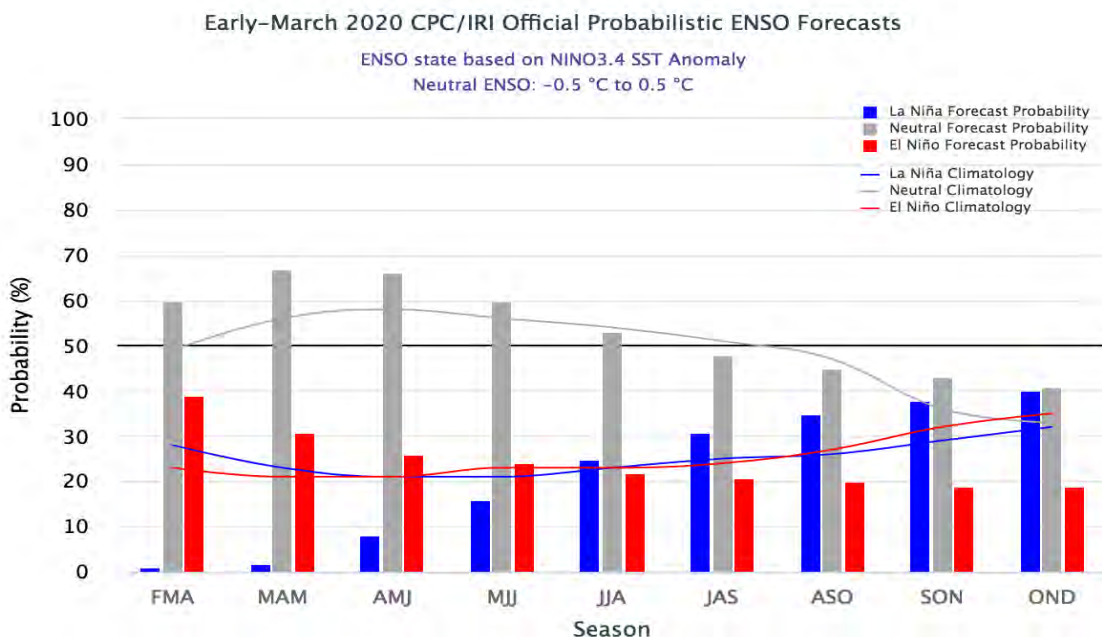
Fuente CPC / IRI Océano PACÍFICO para la Región 3.4 Fig. 2
