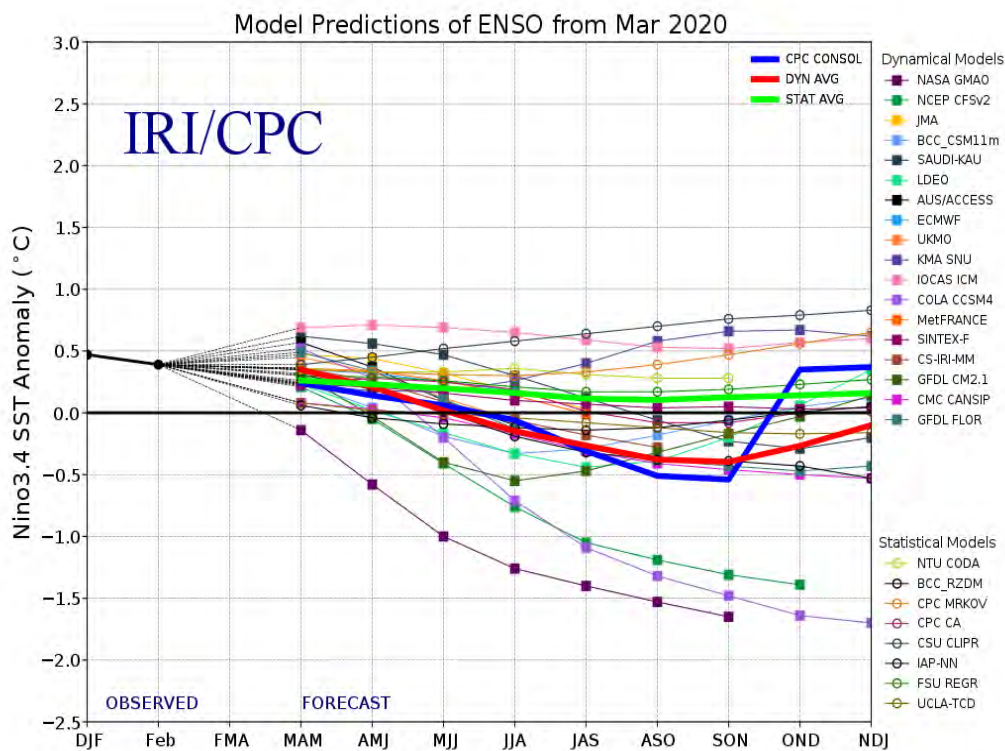
Océano PACÍFICO para la región El Niño / La Niña 3.4 (5°N-5°S, 120°W-170°W) Figura 3.
